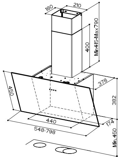
Minimální vzdálenost od varné desky 450 mm.
