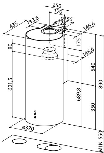
Minimální vzdálenost od varné desky 550 mm .
