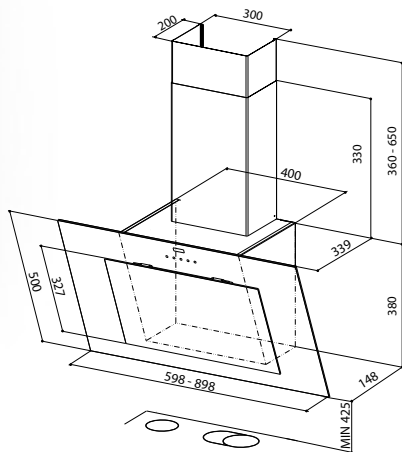
Minimální vzdálenost od varné desky 425 mm.
