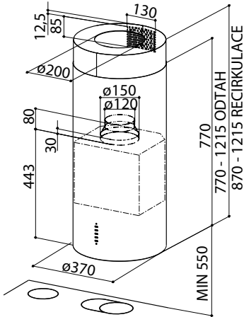
Minimální vzdálenost od varné desky 550 mm.
