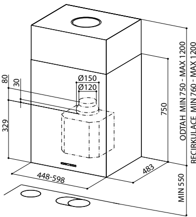
Minimální vzdálenost od varné desky 550 mm.
