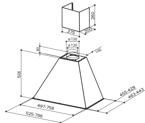
Výška rámu: C1 - 110 mm, C3, C4 - 145 mm
