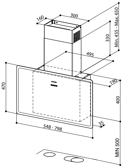
Minimální vzdálenost od varné desky 500 mm.
