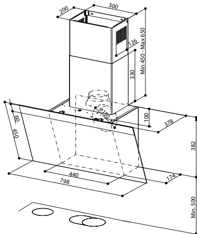
Minimální vzdálenost od varné desky 500 mm.
