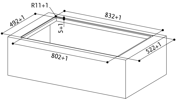
Instalace do roviny s pracovní deskou.
