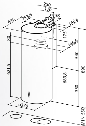
Minimální vzdálenost od varné desky 550 mm .
