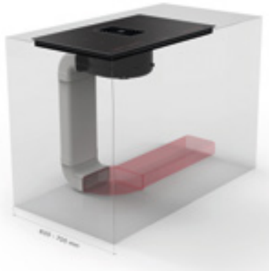
Instalace s výstupem směrem do boku.
