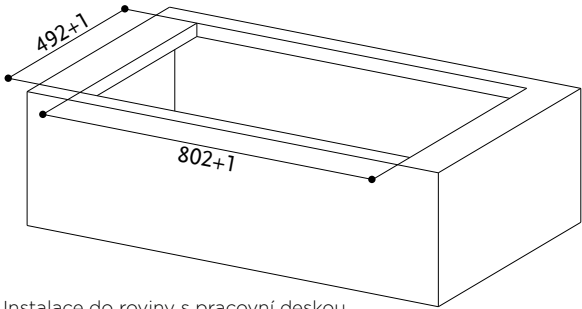
Instalace do roviny s pracovní deskou.
