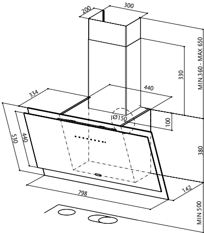
Minimální vzdálenost od varné desky 500 mm.
