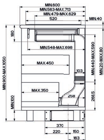
Boční pohled při montáži do 60 cm skříňky
