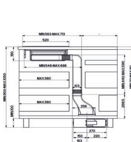
Boční pohled při montáži do ostůvku
